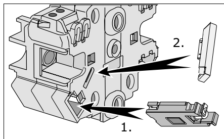
Einsetzen der LED und Lichtleiter Installation de la LED et du conducteur optique Inserimento LED e fotoconduttore
