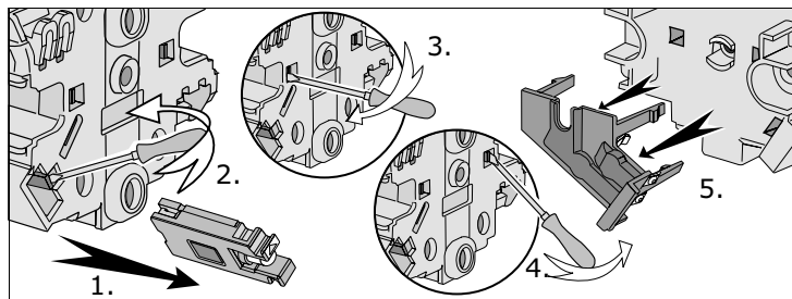
Entfernen des Beleuchtungszusatzes Retrait de l'élément d'éclairage Rimozione aggiunta di illuminazione
